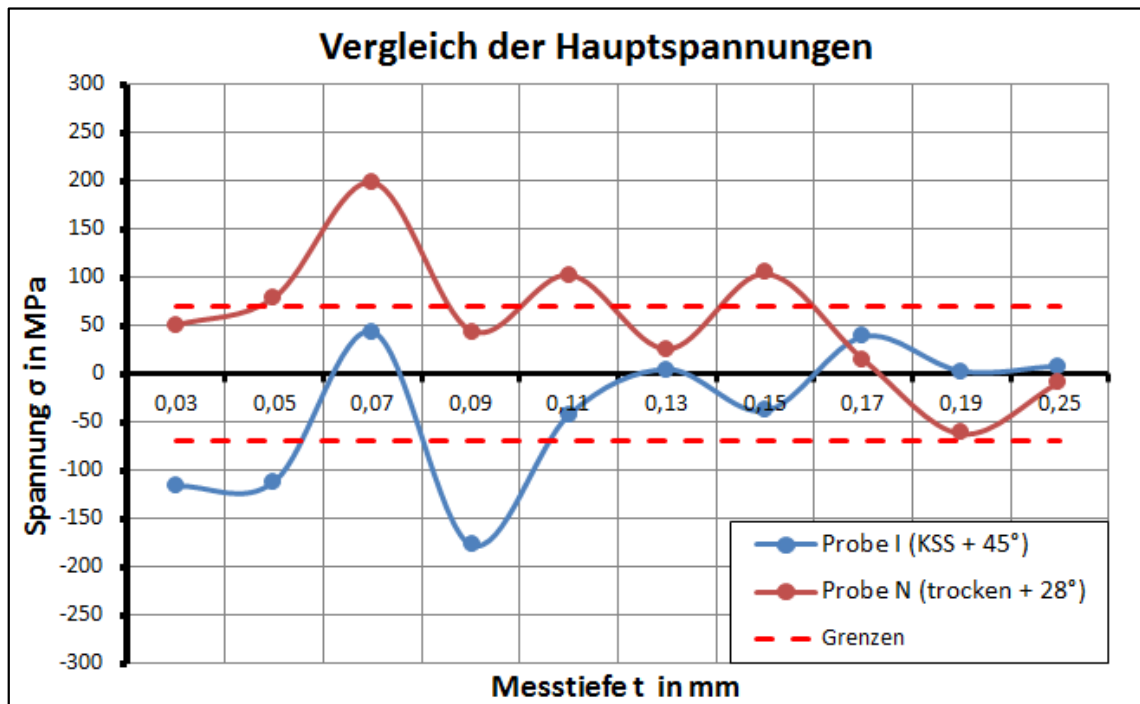
Abbildung 30: Eigenspannungsverläufe im Kombinationsvergleich Kühlung & K_r Proben I und N
