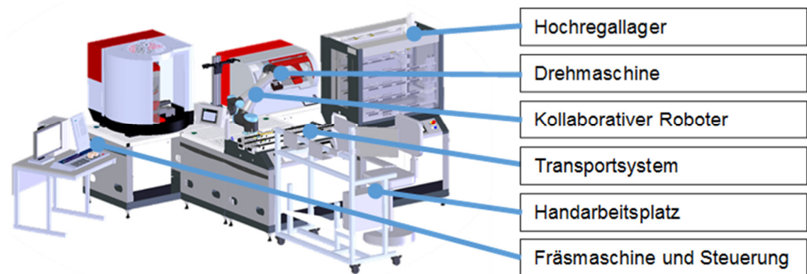
Abbildung 92: Aufbau der Trainingsfabrik 4.0
