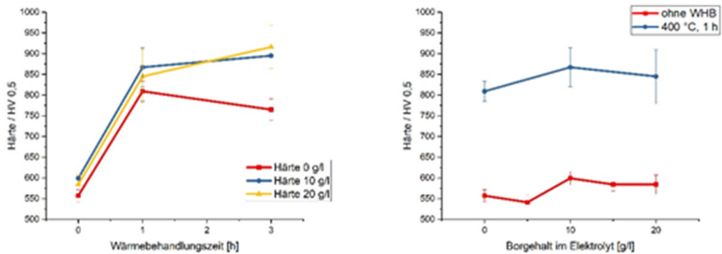
Abbildung 53: Härte der Ni-P-B Schichten bei verschiedene Borgehalte im Elektrolyten und unterschiedliche Wärmebehandlungszeiten
