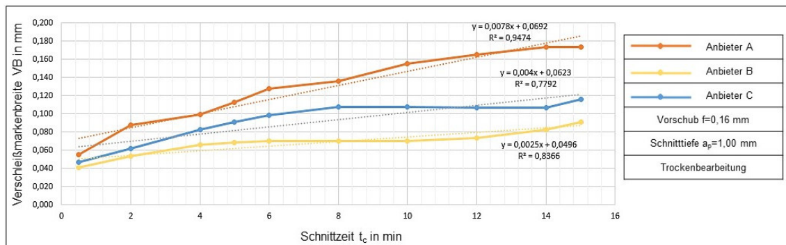
Abbildung 12: Ausbildung der Verschleißmarkenbreite bei v_c = 350 m/min
