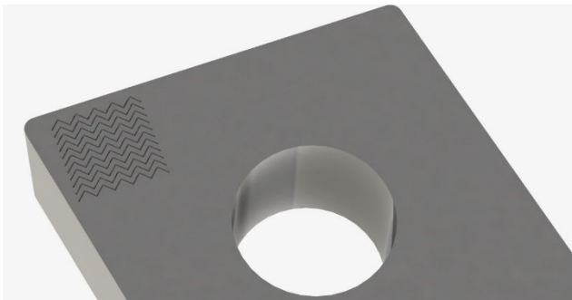
Abbildung 23: Darstellung der Dreieckstruktur
