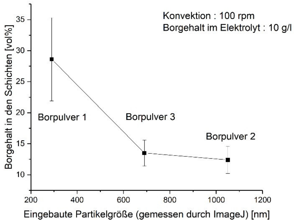
Abbildung 47: Partikeleinbau in den Ni-P-Schichten in Abhängigkeit der durch ImageJ gemessene Größe der eingebauten Borpartikel
