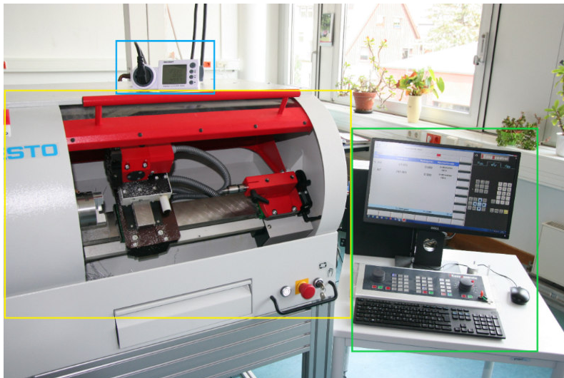
Abbildung 62 Versuchsaufbau EMCO CT60 [50]
