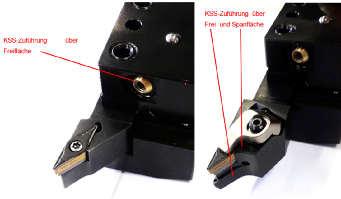
Abbildung 18: Drehwerkzeuge für KSS-Zuführung
