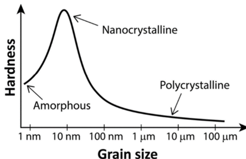
Abbildung 54: Zusammenhang zwischen der Korngröße und der Härte eines Materials
