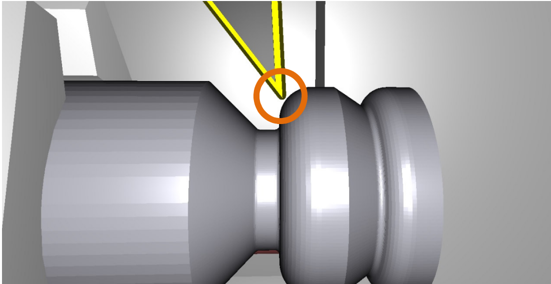
Abbildung 91: Durch fehlerhaftes NC-Programm entstandener Versatz zwischen Werkzeug und Werkstück
