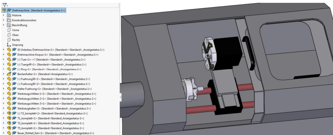
Abbildung 81: Aufgebautes Gesamtmodell der Wabeco CC-D 100 in CAD
