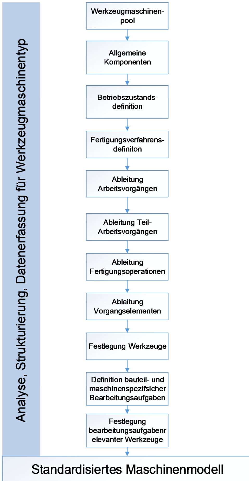
Abbildung 121: Vorgehen zur Entwicklung eines Standardisierten Maschinenmodells
