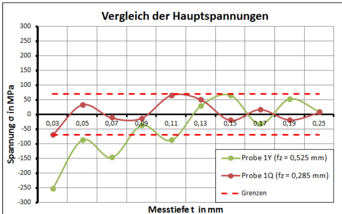
Abbildung 36: Ausgewerteten Tiefenverläufe Probe 1Y und 1Q
