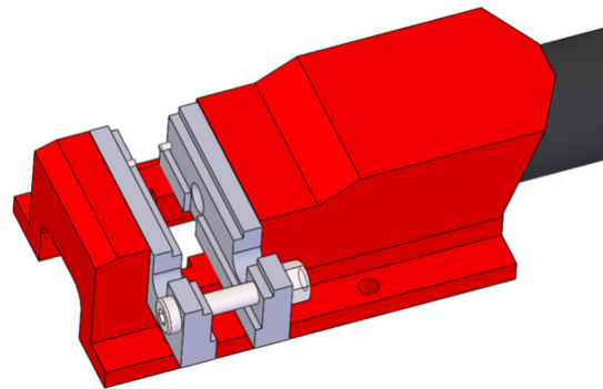
Abbildung 114: Zusätzlich gefertigte Spannbacken (grau) im Maschinenschraubstock (rot)
