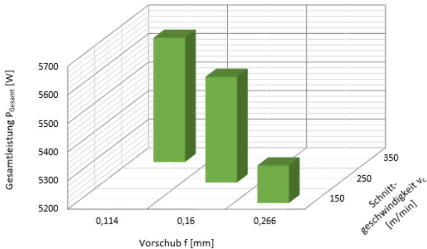
Abbildung 21: Vergleich der Versuche bei konstantem Zeitspannvolumen
