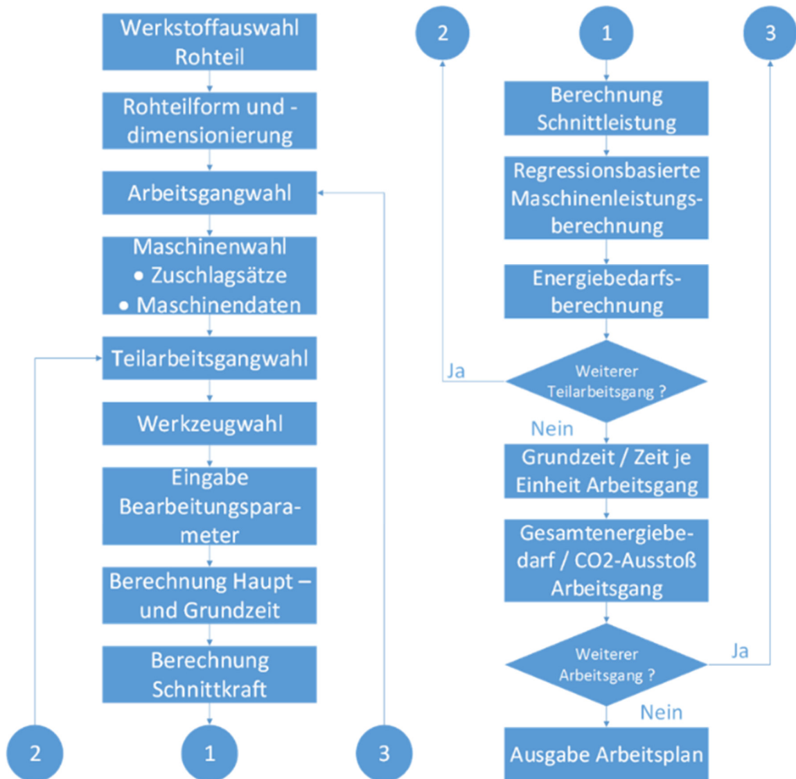
Abbildung 72: Ablaufdiagramm des Planungsprozesses [51]
