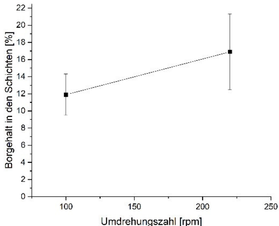
Abbildung 50: Einfluss der Hydrodynamik des Elektrolyten an dem Partikeleinbau in den Ni-P Schichten
