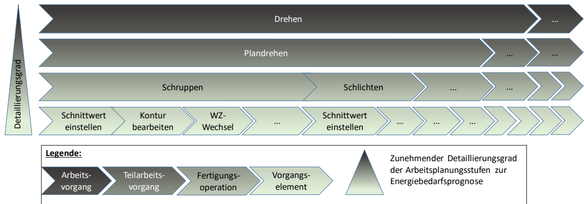
Abbildung 64: Prozessstruktur für Datenaufnahme an EMCO CT60 i.A.a. [80]
