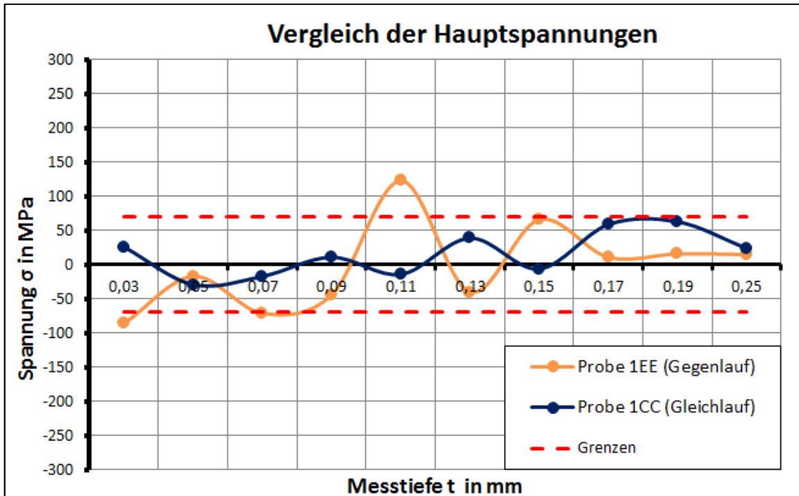
Abbildung 34: Ausgewerteten Tiefenverläufe Probe 1EE und 1CC
