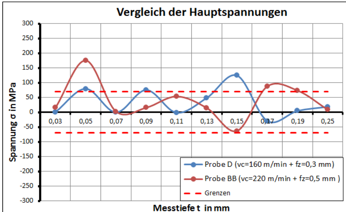
Abbildung 28: Eigenspannungsverläufe im Kombinationsvergleich v_c und f_z Proben D und BB
