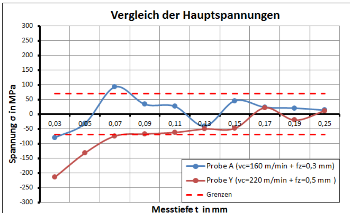
Abbildung 29: Eigenspannungsverläufe im Kombinationsvergleich v_c und f_z Proben A und Y
