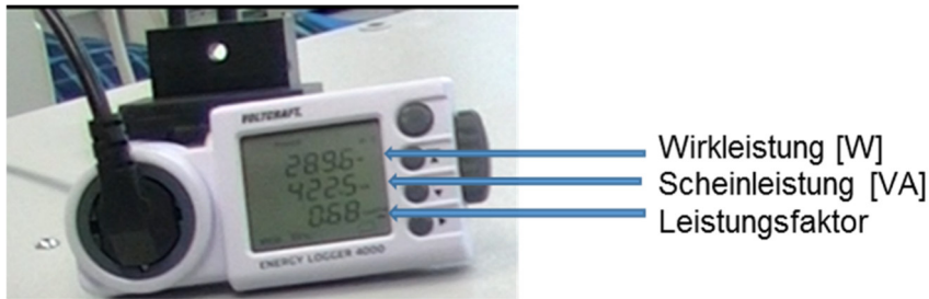
Abbildung 63: Messgerät
