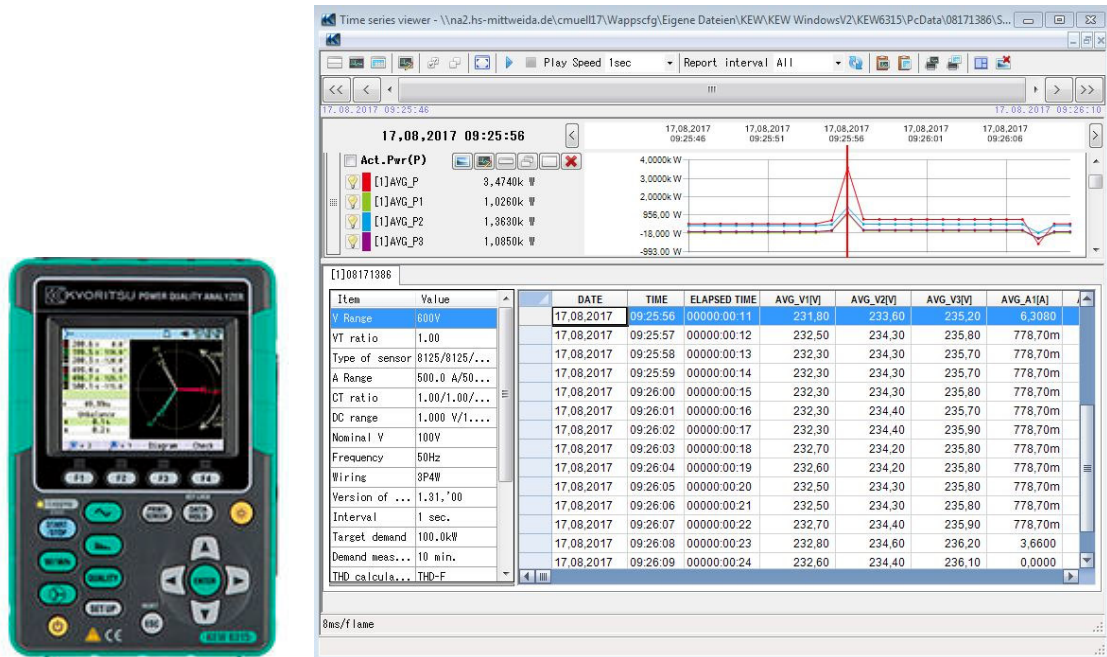
Abbildung 68: Messgerät KEW 6315 und zugehöriger Software [51]
