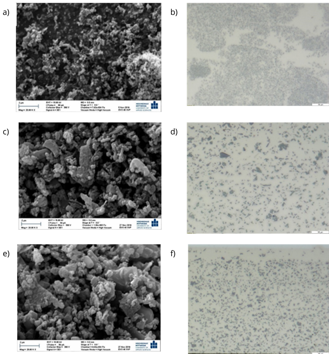
Abbildung 46: REM-Aufnahme (20 000x Vergrößerung) von a) Borpulver 1, b) Borpulver 2, c) Borpulver 3 und die metallographische Querschliffe der Ni-P-B-Schichten (100x Vergrößerung) mit b) Borpulver 1, d) Borpulver 2 und f) Borpulver 3
