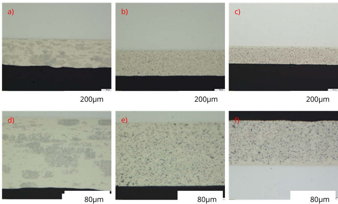
Abbildung 48: Die metallographische Querschliffe bei 20x und 50x Vergrößerung für Ni-P-B Schichten mit eingebauten Borpulvern a) d) Pulver 1, b) e) Pulver 2, und c) f) Pulver 3
