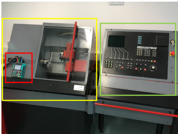
Abbildung 69: Versuchsaufbau [51]
