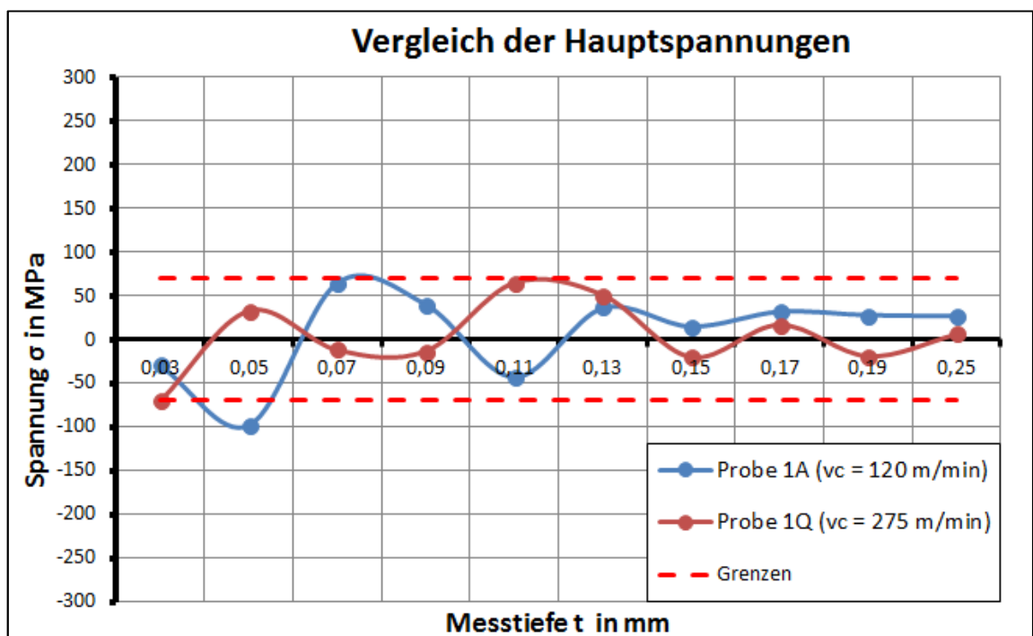
Abbildung 37: Ausgewerteten Tiefenverläufe Probe 1A und 1Q
