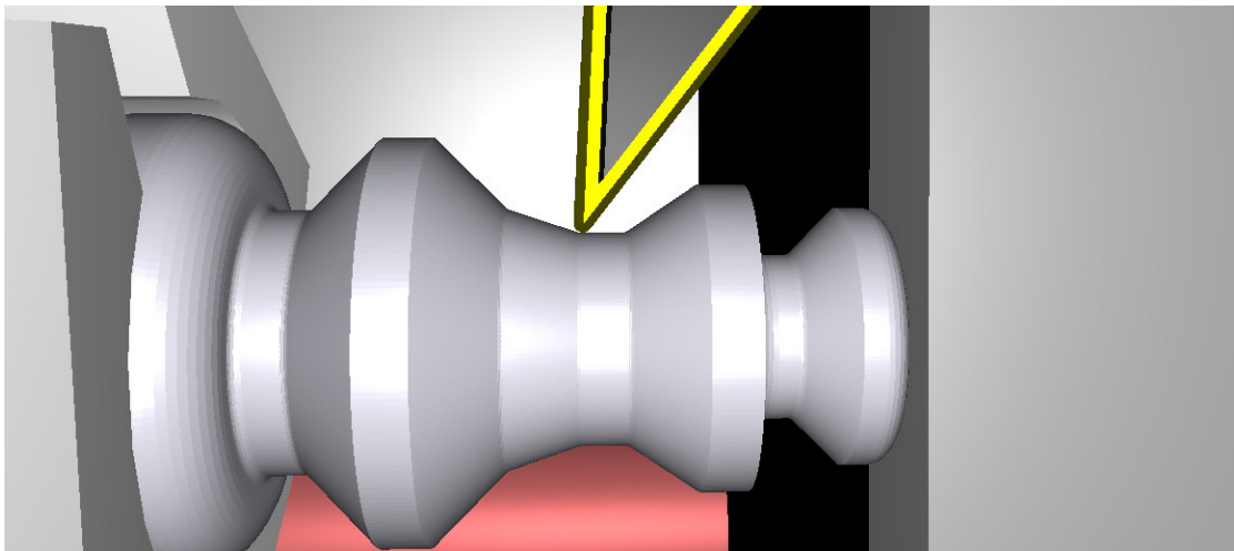
Abbildung 90: Exakt arbeitende Maschinensimulation
