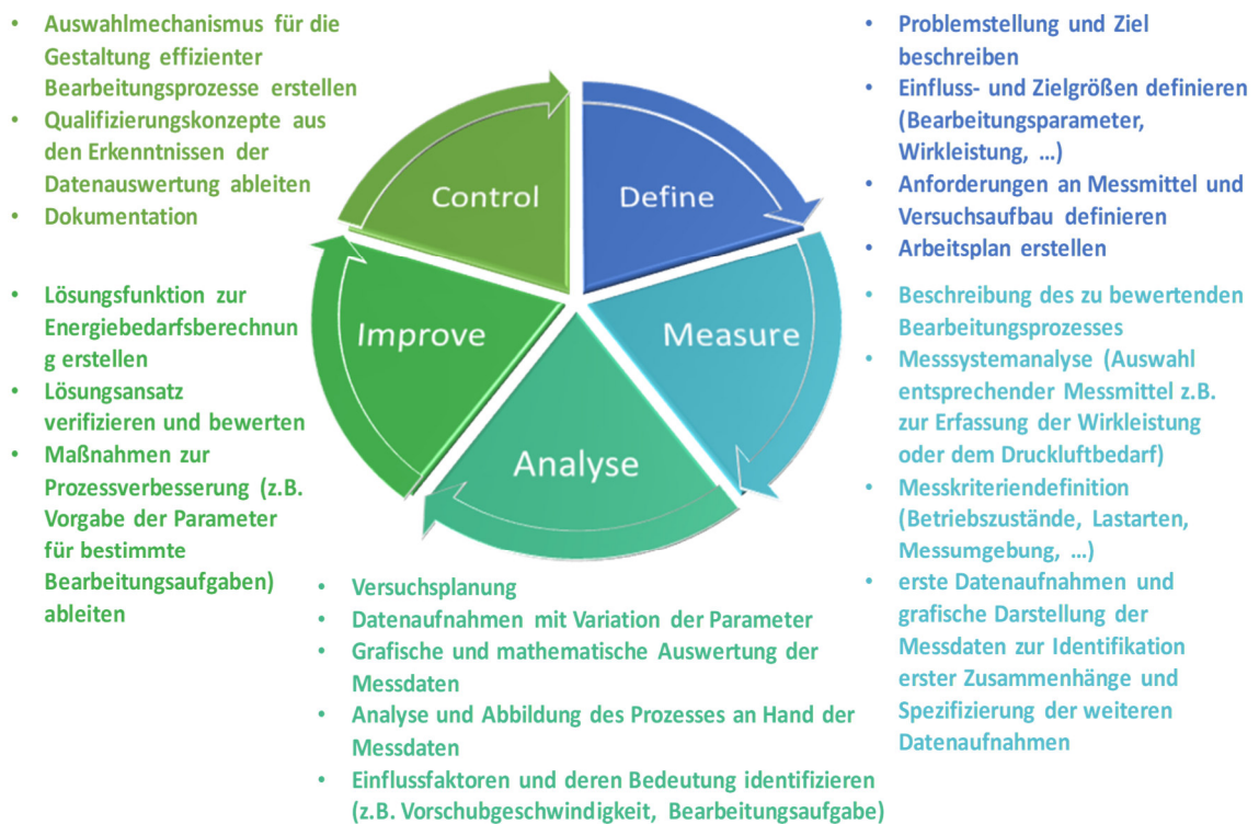
Abbildung 60: DMAIC-Zyklus für die Leistungsmessung und Datennutzung i.A.a. [48]
