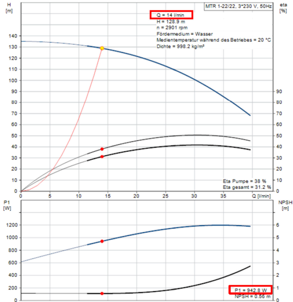
Abbildung 77: Leistungskennlinie von Hydraulikpumpe [56]
