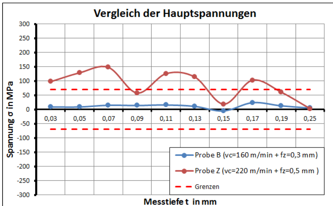
Abbildung 27: Eigenspannungsverläufe im Kombinationsvergleich v_c und f_z Proben B und Z
