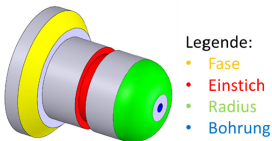
Abbildung 61: Referenzbauteil für Messungen an den Referenzmaschinen [51]
