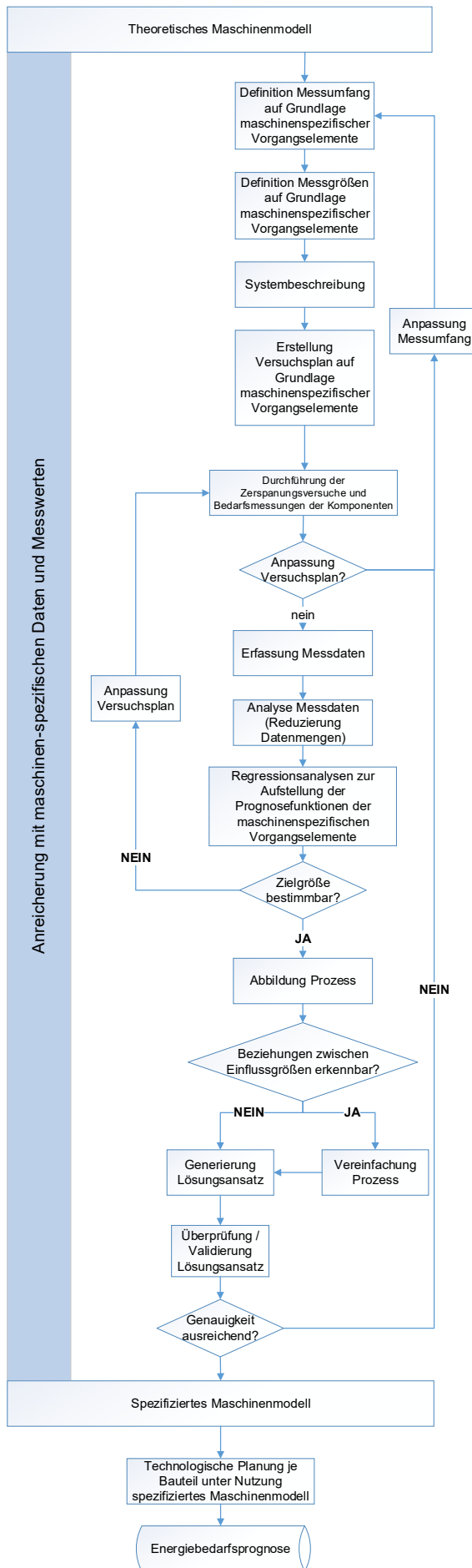
Abbildung 123: Vorgehen zur Entwicklung eines Spezifizierten Maschinenmodells
