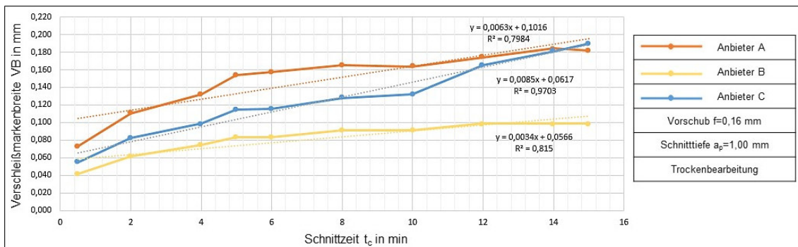
Abbildung 11: Ausbildung der Verschleißmarkenbreite bei v_c = 250 m/min
