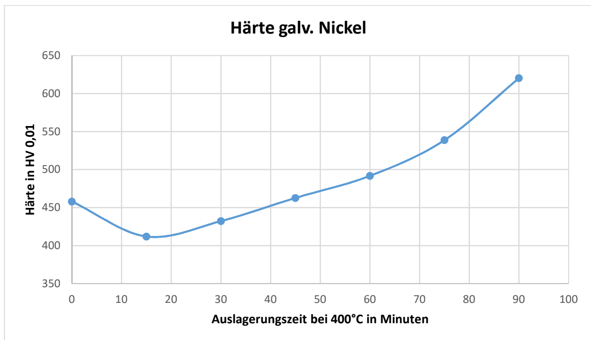
Abbildung 41: Einfluss der Wärmebehandlung auf die Härte Ni-B-Schichten
