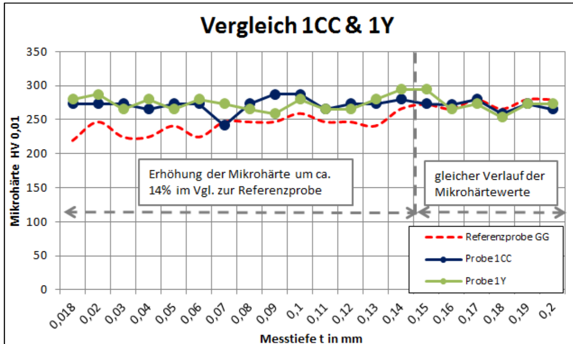
Abbildung 39: Darstellung der Mikrohärteverläufe Proben CC und Y
