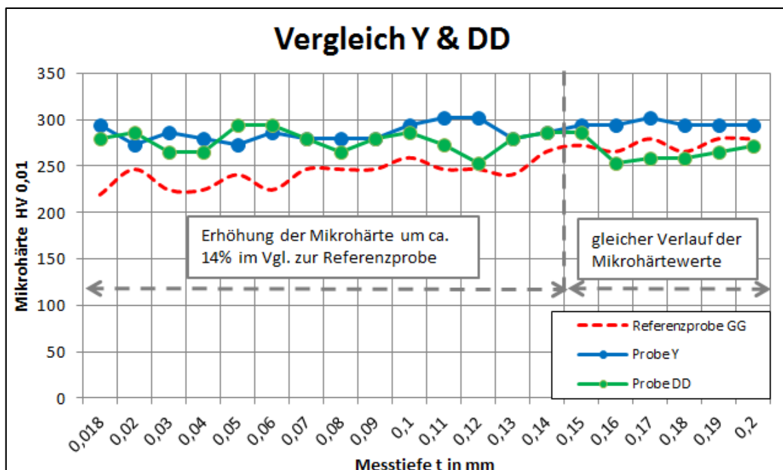
Abbildung 38: Darstellung der Mikrohärteverläufe Proben Y und DD
