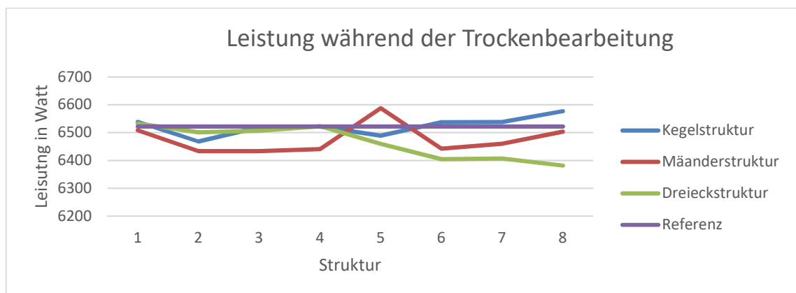
Abbildung 25: Leistung während der Trockenbearbeitung
