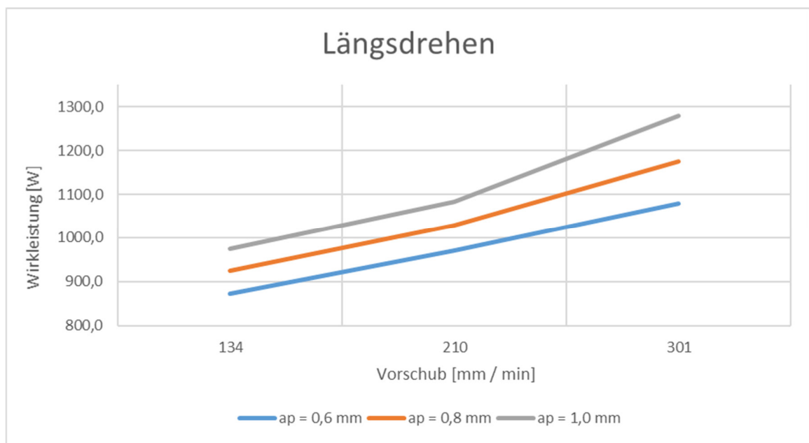
Abbildung 70: Leistungsbedarf Längsdrehen (graphisch) [51]
