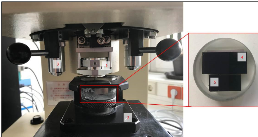
Abbildung 26: Versuchsaufbau der Mikrohärtprüfung
