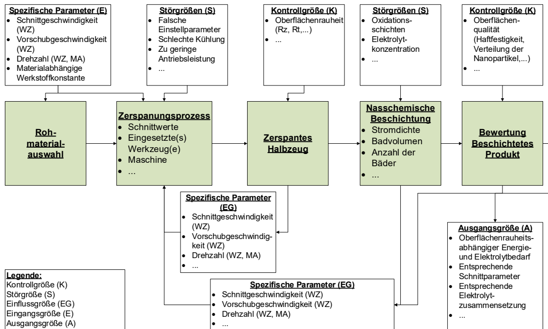
Abbildung 116: Regelkreis zur ressourcenorientierten Fertigung hochbeanspruchter Bauteile
