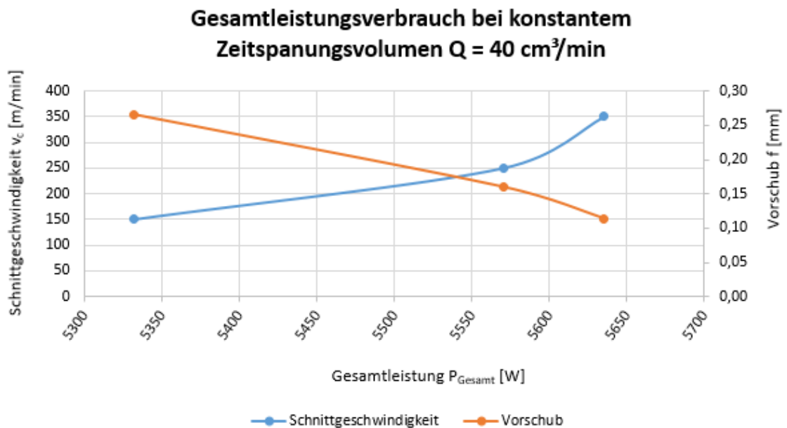
Abbildung 20: Gesamtleistungsbedarf bei konstantem Zeitspannvolumen
