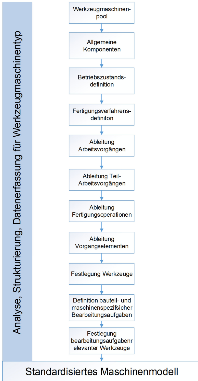
Abbildung 58: Standardisiertes Maschinenmodell
