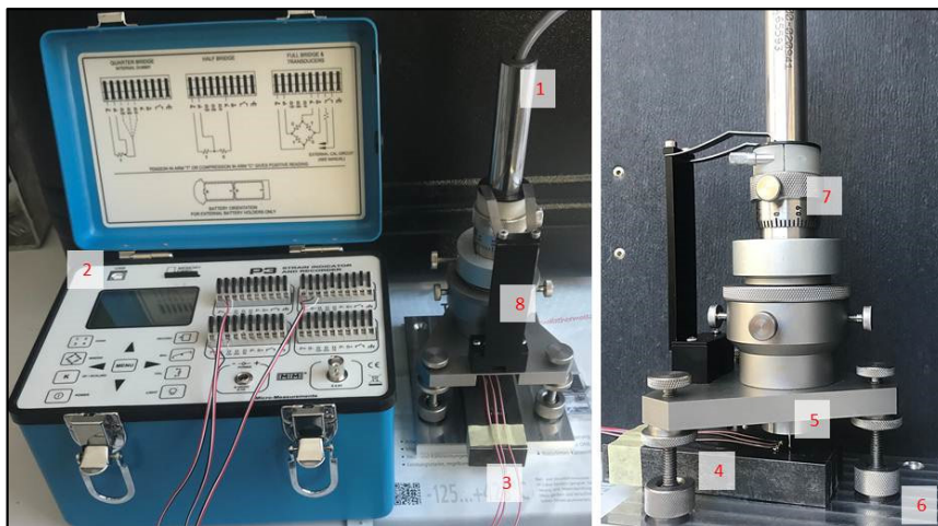
Abbildung 24: Versuchsaufbau der Eigenspannungsmessungen
