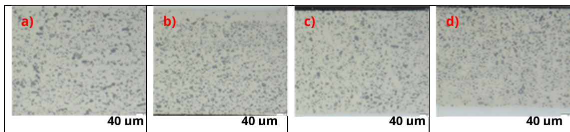
Abbildung 52: Metallographische Querschliffe bei 100x Vergrößerung für Partikelgehalt im Elektrolyten von a) 5 g/l, b) 10 g/l, c) 15 g/l und d) 20 g/l
