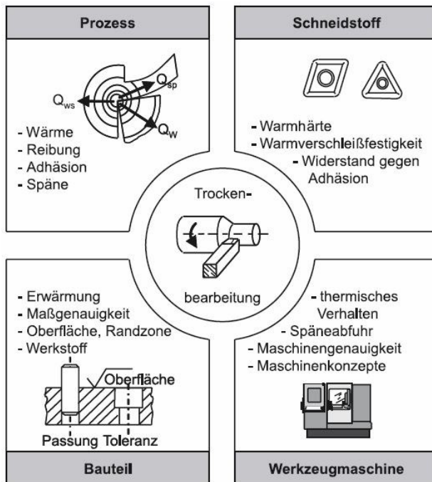
Abbildung 7: Anforderungen an die Trockenbearbeitung [24]
