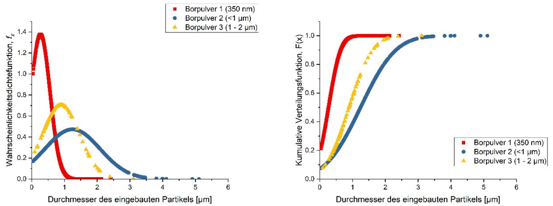
Abbildung 45: Verteilung der Borpartikel in den Ni-P-Schichten
