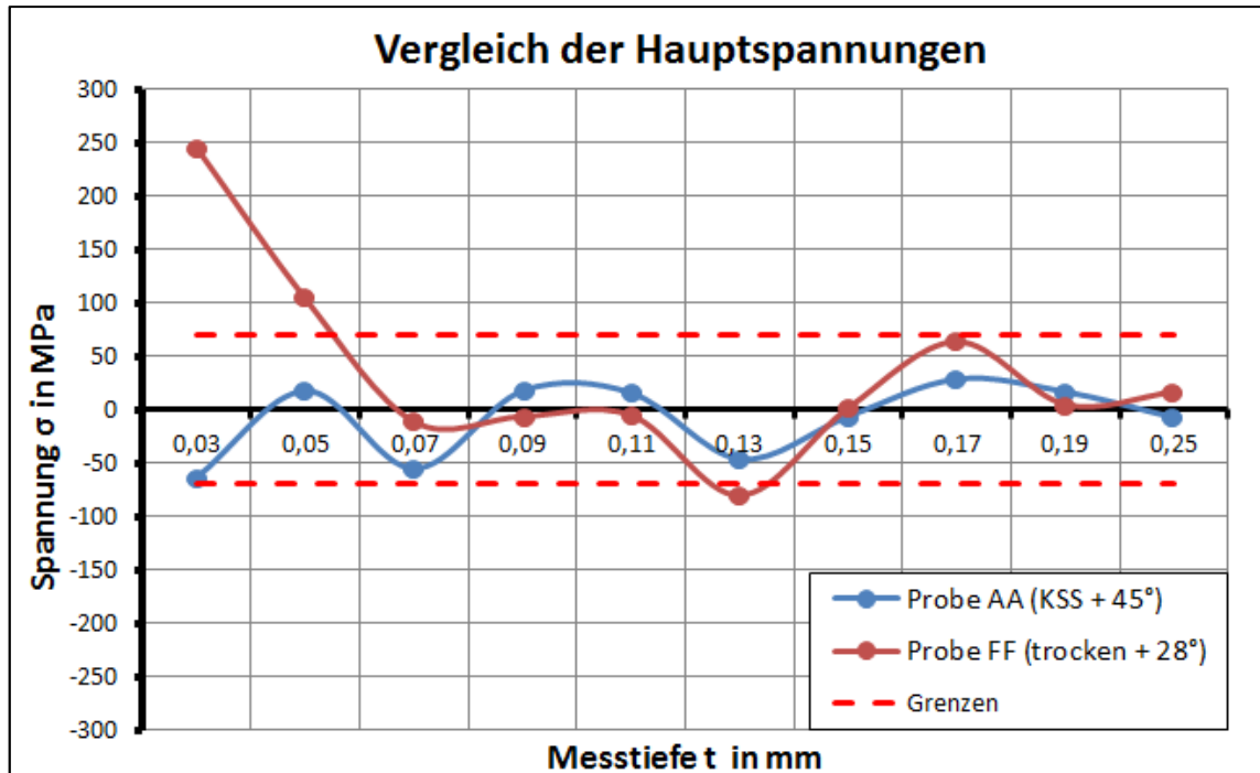
Abbildung 31: Eigenspannungsverläufe Kombinationsvergleich Kühlung & K_r Proben AA und FF
