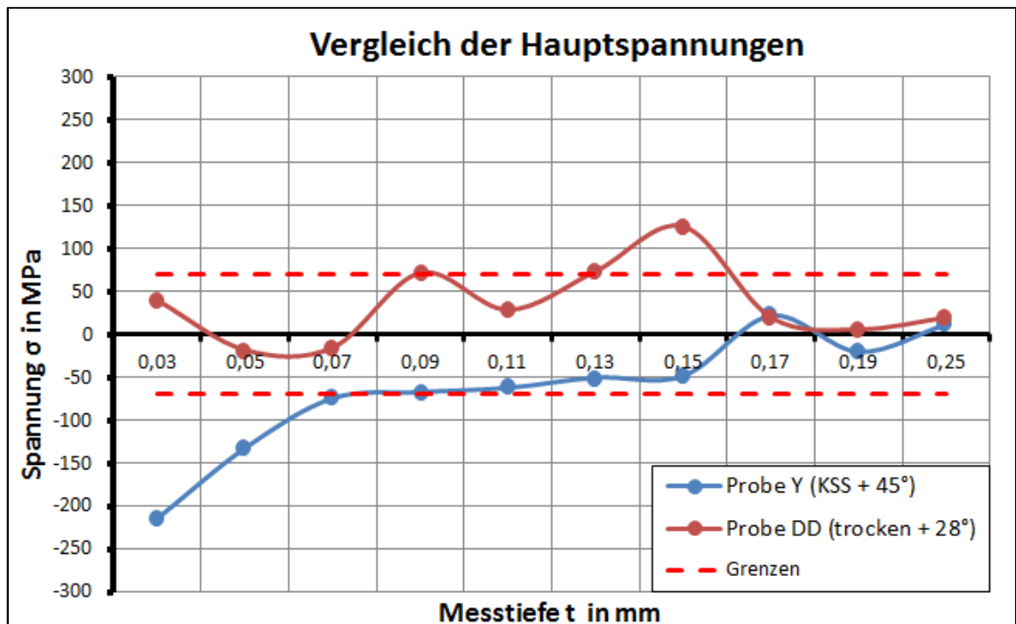
Abbildung 32: Eigenspannungsverläufe Kombinationsvergleich Kühlung & K_r Proben Y und DD
