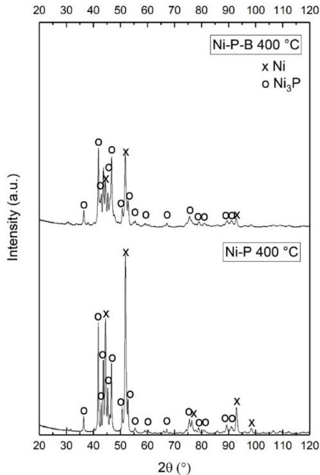
Abbildung 56: XRD Diffraktogramm von Ni-P und Ni-P-B Schichten bei 400 °C und 3 h
