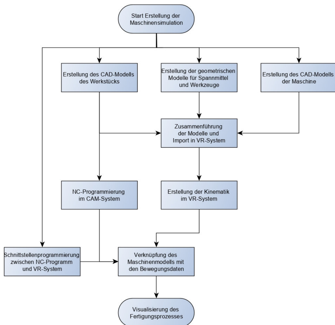
Abbildung 78: Ablaufplan zur Erstellung einer Maschinensimulation
