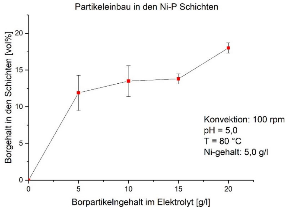
Abbildung 51: Partikeleinbau in den Ni-P-Schichten in Abhängigkeit des Partikelgehalts im Elektrolyten
