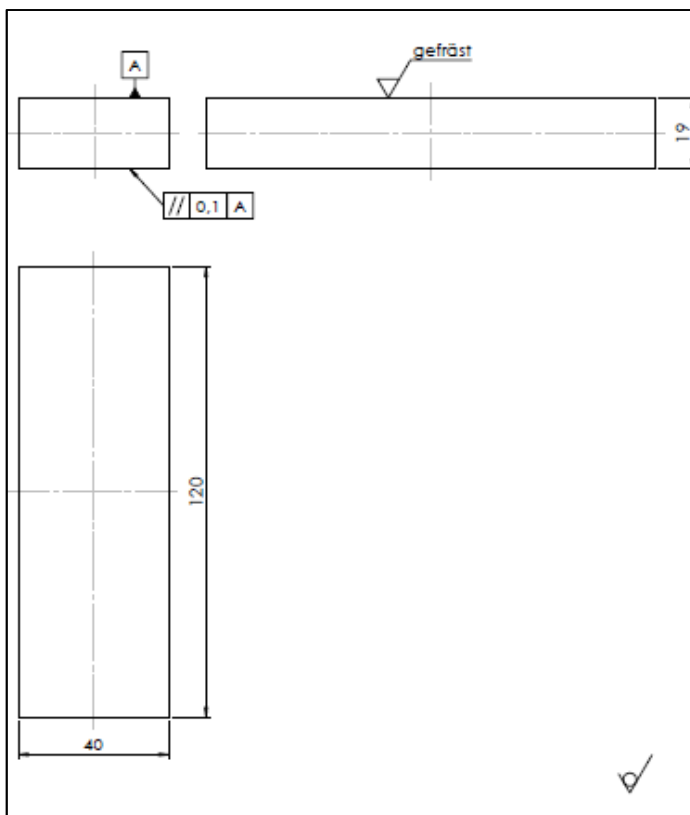
Abbildung 23: Probengeometrie
