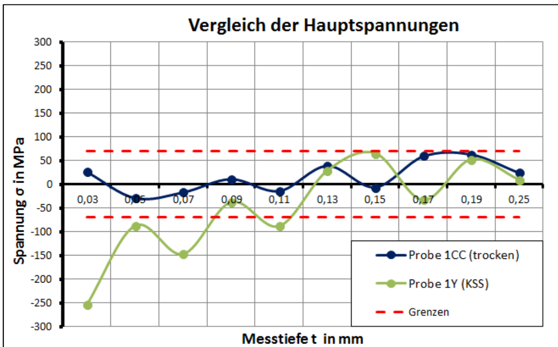
Abbildung 35: Ausgewerteten Tiefenverläufe Probe 1CC und 1Y
