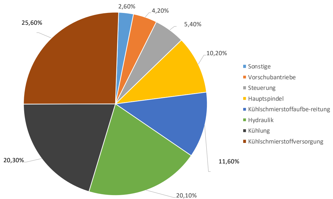
Abbildung 74: Typische Energiebedarfsaufteilung von Werkzeugmaschinen nach [54]
