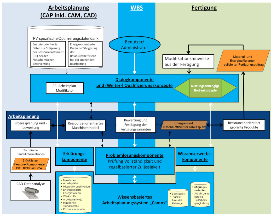
Abbildung 115: Modell zur ganzheitlichen ressourceneffizienten Produktion
