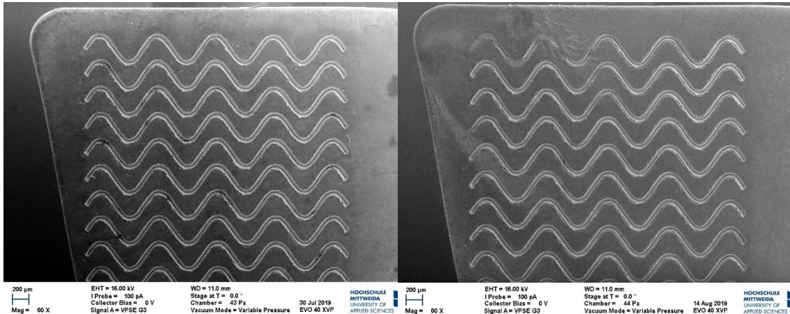
Abbildung 27: Wendeschneidplatte vor der Trockenbearbeitung
