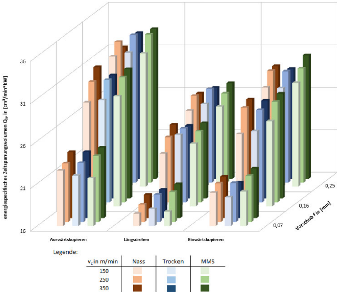
Abbildung 17: Vergleich der Abschnitte Musterwelle
