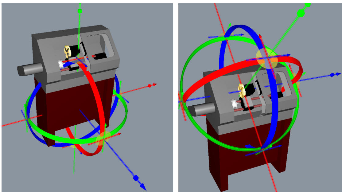
Abbildung 86: Änderung der Koordinatensystemposition am Beispiel des Werkzeughalters
