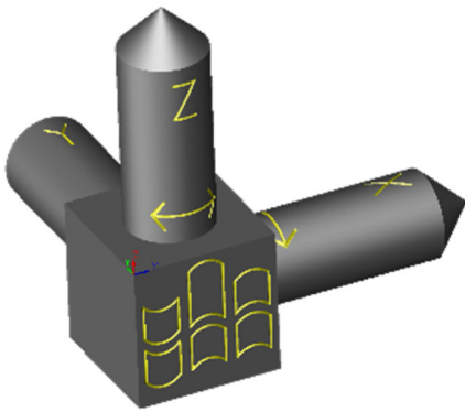
Abbildung 113: Beispielbauteil "Koordinatensystem" in der Musterlösung
