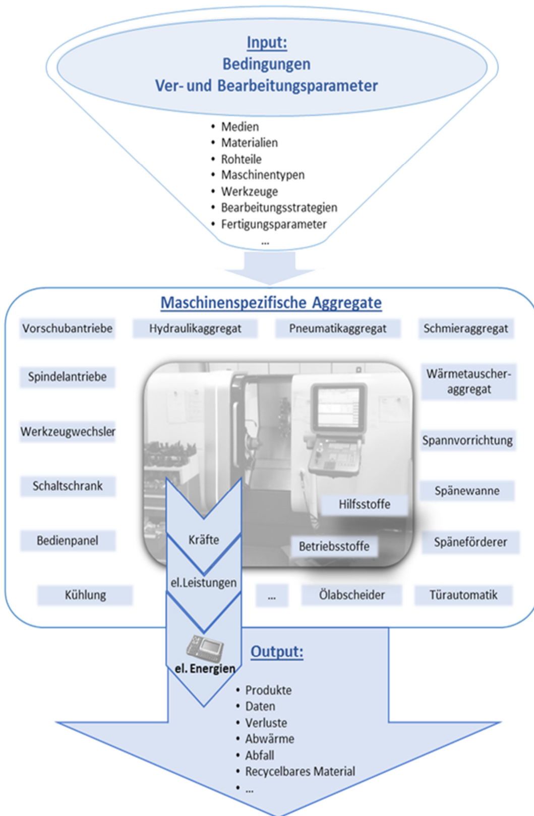
Abbildung 59: Theoretisches Maschinenmodell am Beispiel DMG Mori CTX Alpha 500
