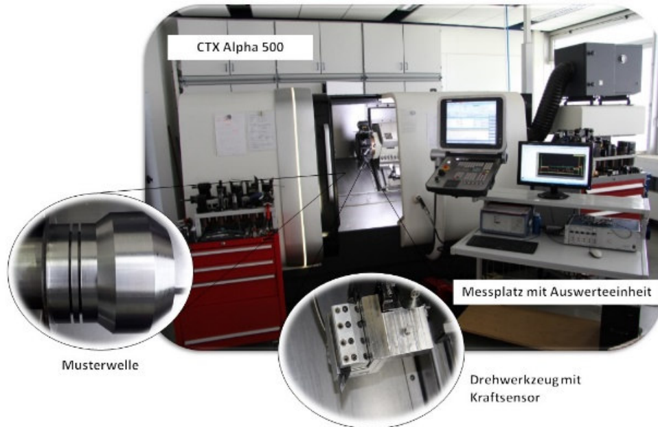
Abbildung 4: Werkzeugmaschine CTX Alpha 500
