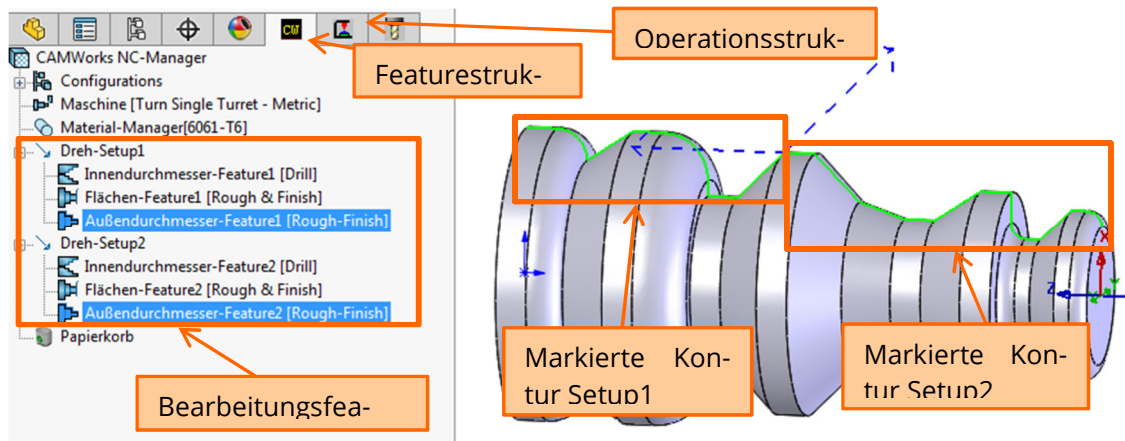
Abbildung 84: Vollständiger „Arbeitsplan“ für die Schachfigur Bauer
