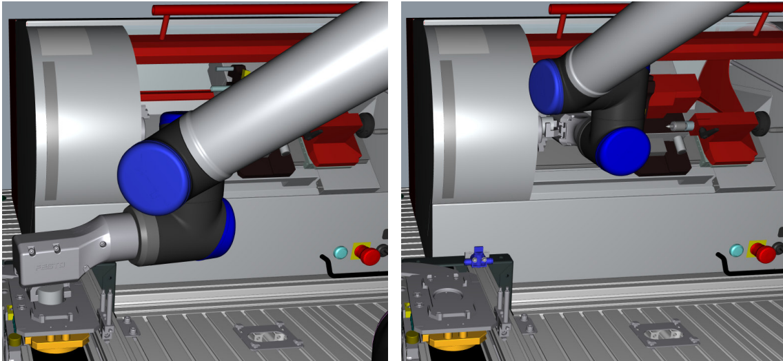
Abbildung 94: Beschickung eines Werkstücks vom Transportband (links) zur Drehmaschine (rechts)
