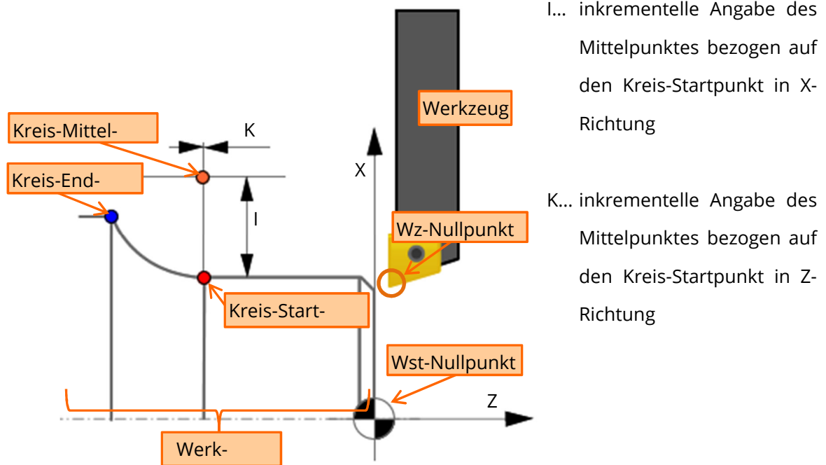
Abbildung 85: Darstellung I- und K-Adresse am Beispiel G02-Befehl i.A.a [55]; [64]
