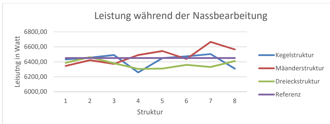
Abbildung 26: Leistung während der Nassbearbeitung
