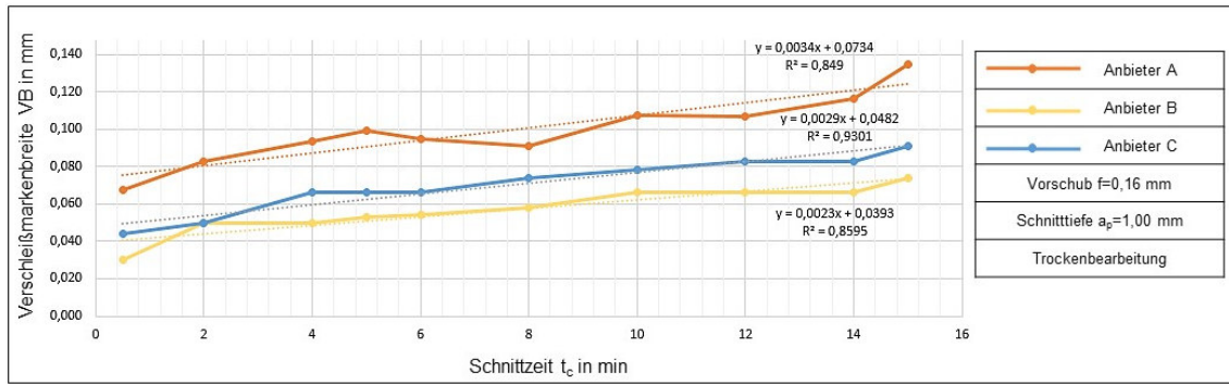
Abbildung 10: Ausbildung der Verschleißmarkenbreite bei v_c = 150 m/min
