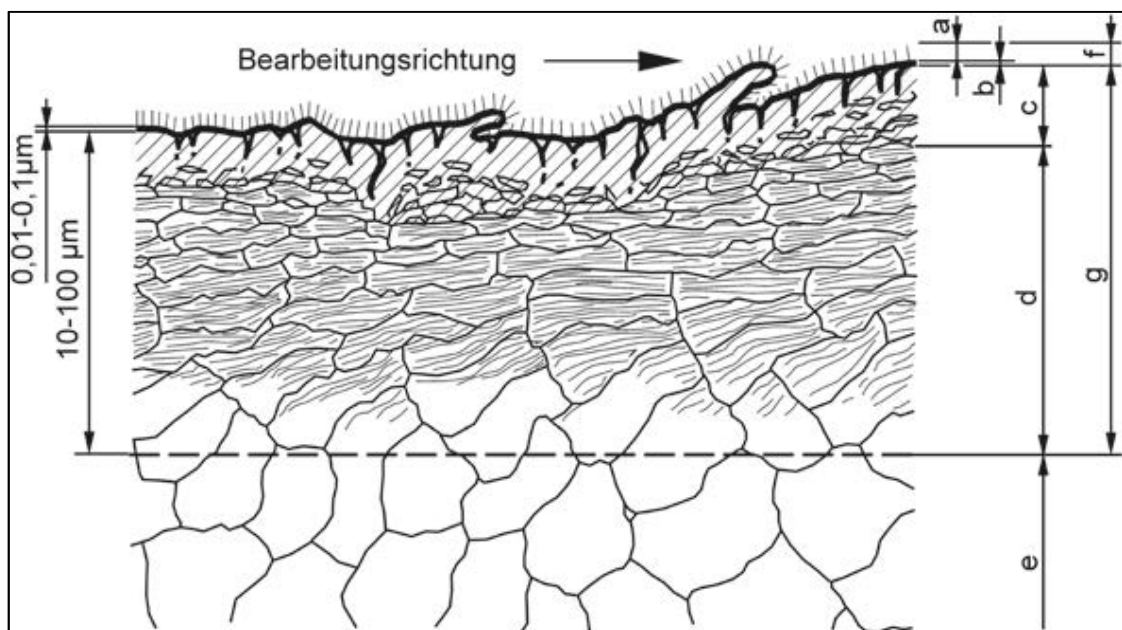
Abbildung 22: Schematische Darstellung der Bauteilrandschicht nach [1]
