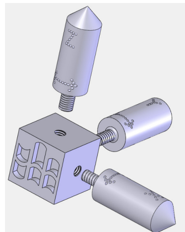
Abbildung 109: Beispielbauteil, konstruktiv neu gestaltet für alternative Ansätze hinsichtlich Rohmaterials und Fertigungsverfahren zur Umsetzung des Qualifizierungskonzeptes
