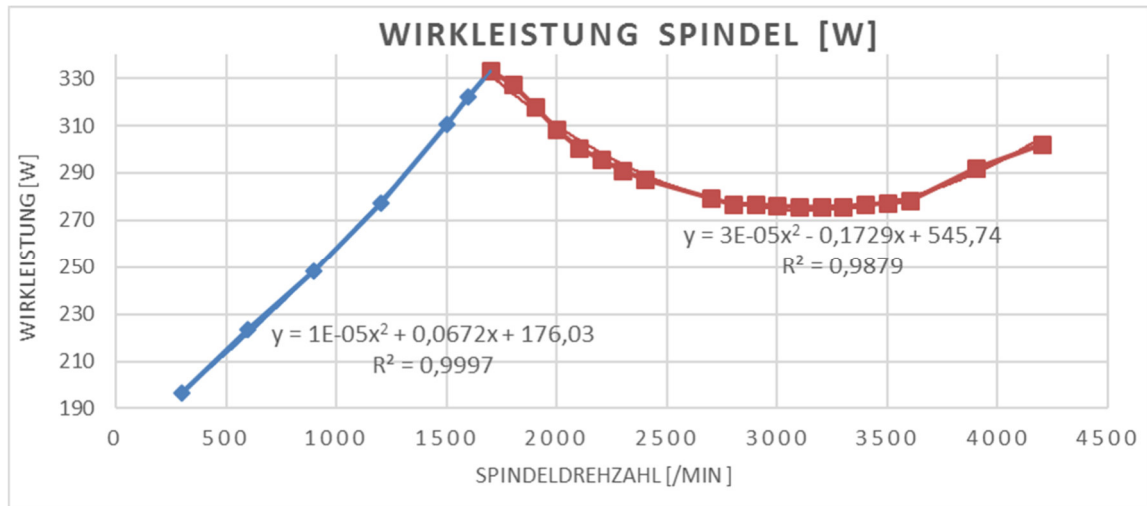
Abbildung 66: Regressionsanalyse zur graphischen Darstellung des Leistungsbedarfs Spindel EMCO CT60 [50]
