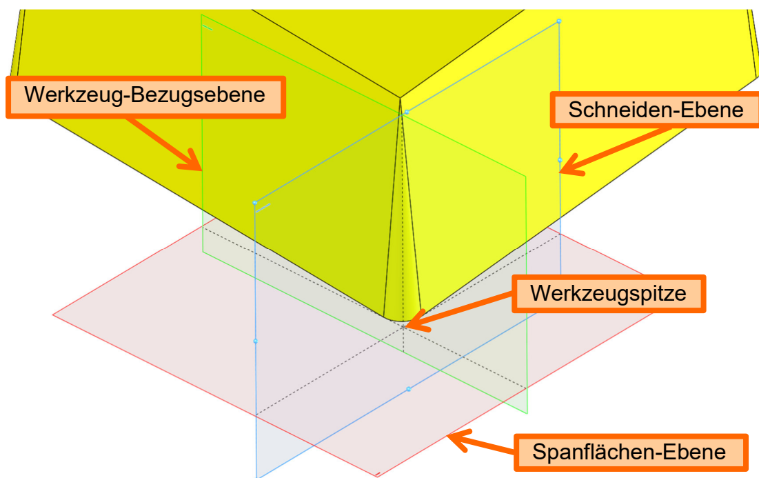
Abbildung 80: Ebenen-Beziehungen und Werkzeugspitze an einer Wendeschneidplatte [62]
