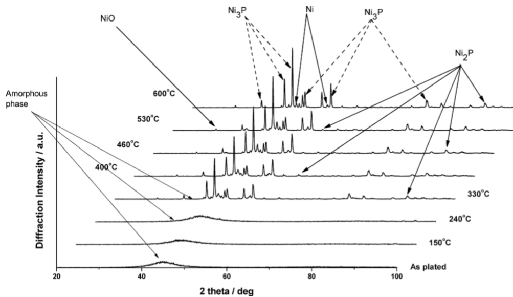
Abbildung 55: XRD Diffraktogramm von Ni-P Schichten bei verschiedene Wärmebehandlungs-temperaturen
