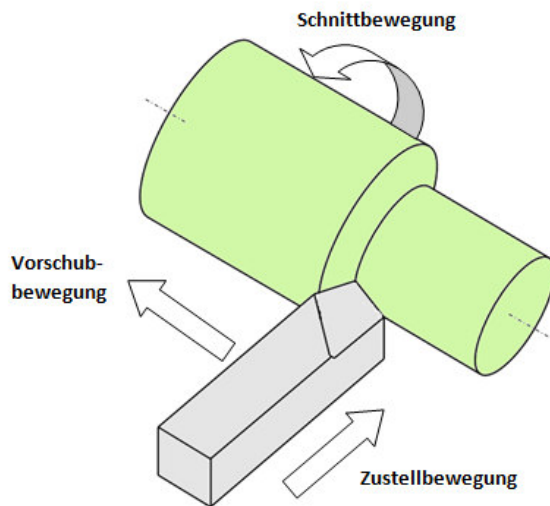
Abbildung 3: Arbeitsbewegungen beim Fertigungsverfahren Drehen
