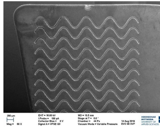
Abbildung 30: Wendeschneidplatte nach der Nassbearbeitung
