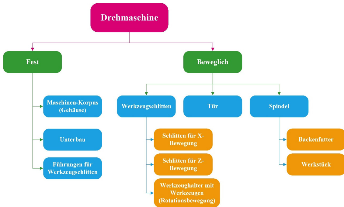
Abbildung 82: Komponentenbaum des Gesamtmodells
