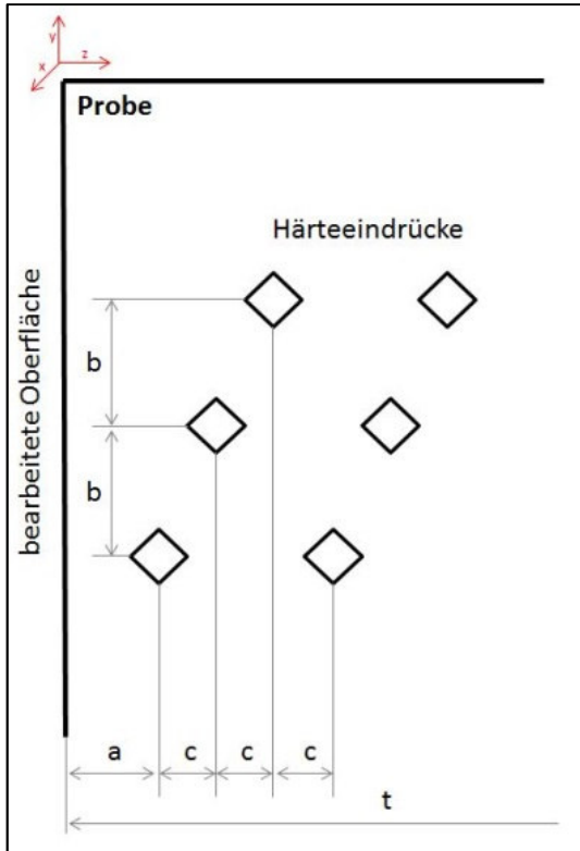
Abbildung 25: Schematische Darstellung zum Vorgehen der Mikrohärtprüfung
