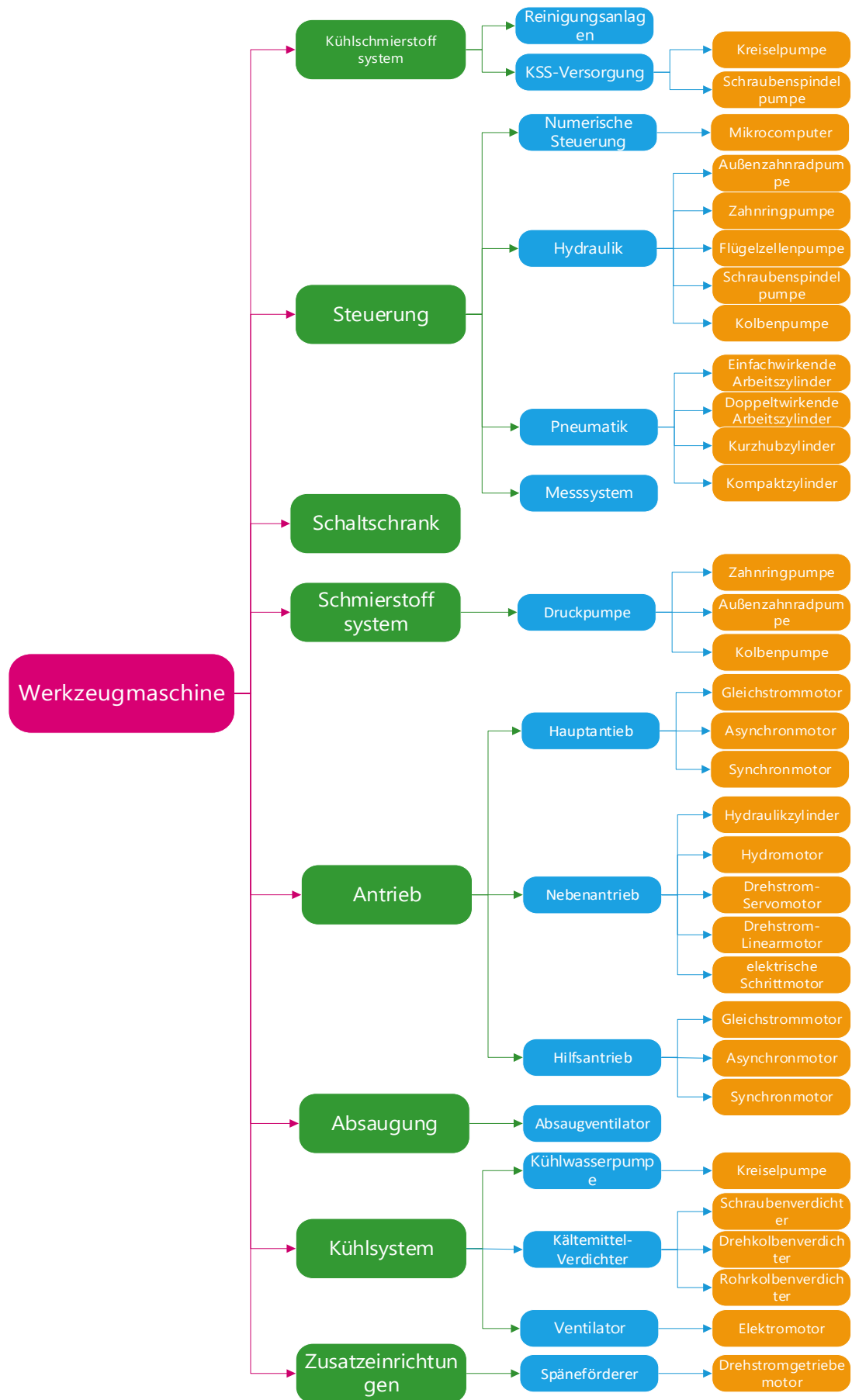
Abbildung 75: Komponentenbaum allgemeine Werkzeugmaschine [92]
