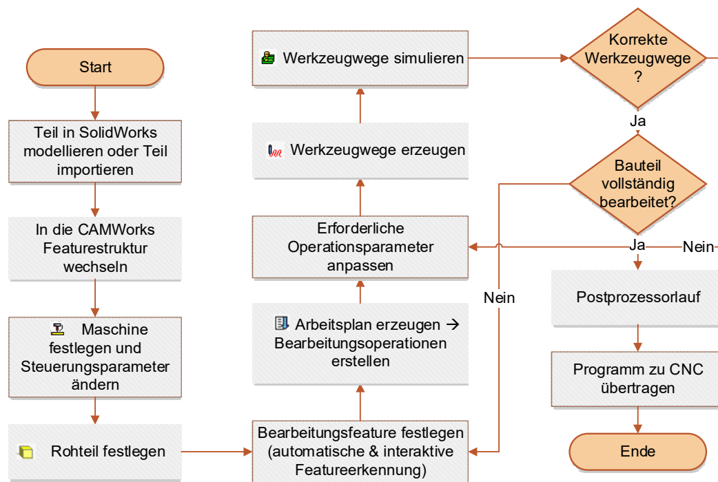
Abbildung 83: CAMWorks- Ablaufdiagramm i.A.a. [61]
