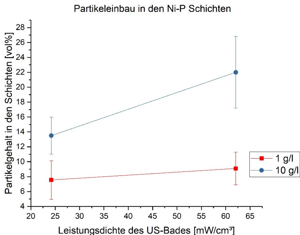
Abbildung 49: Der Partikeleinbau in den Ni-P-Schichten unter den Einfluss des Ultraschalls mit verschiedene Leistungsdichte
