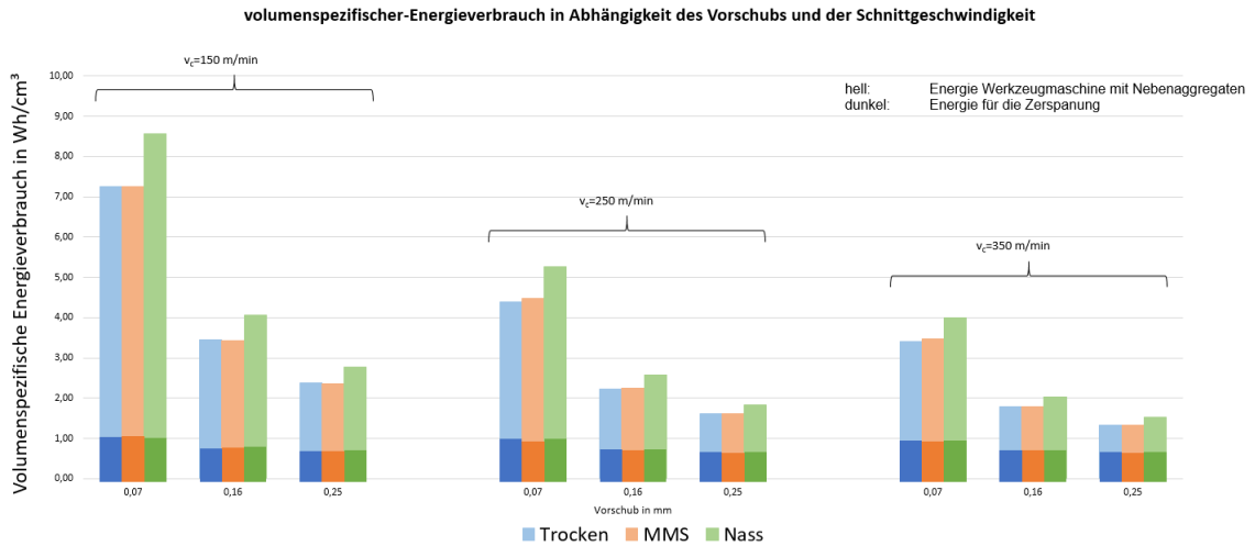
Abbildung 16: Energiebedarf bezogen auf das abgespannte Volumen
