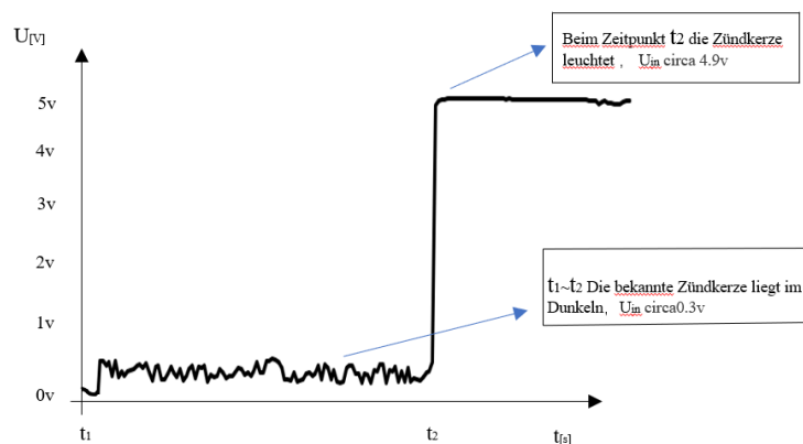
Abbildung 6: analoges Spannungssignal im Pin A0
