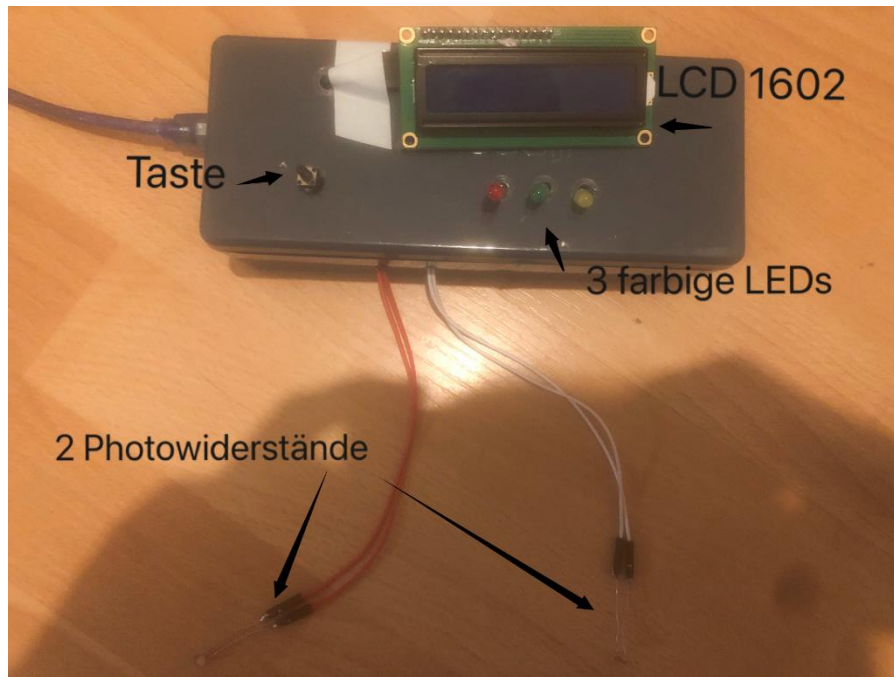
Abbildung 19: Aufbau von System
