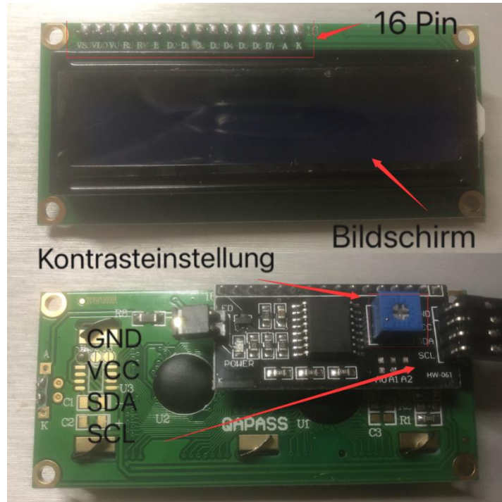
Abbildung 9: Beispiel von LCD 1602 und I2C/SPI LCD
