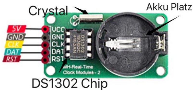
Abbildung 10: DS 1302 Modul[6]
