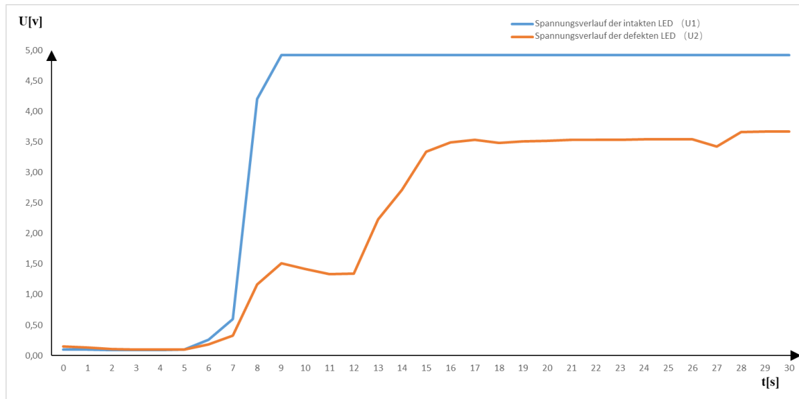
Abbildung 25: Spannungsverläufer der intakte LED (U1) und defekte LED (U2) beim Fall 2
