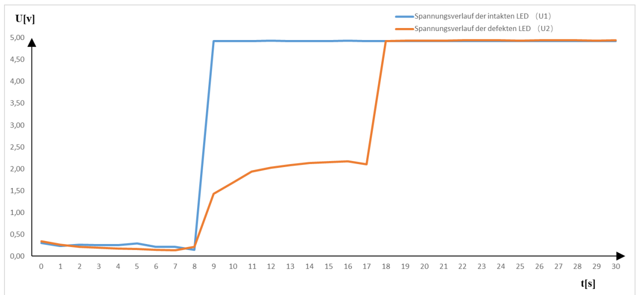
Abbildung 22: Spannungsverläufer der intakten LED (U1) und defekte LED (U2) beim Fall 1
