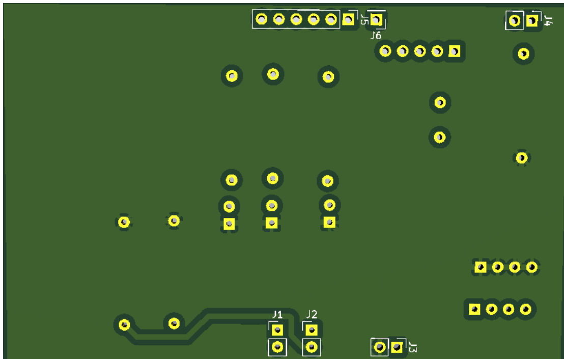
Abbildung 35: Abbildung 31: PCB(Rückseite)
