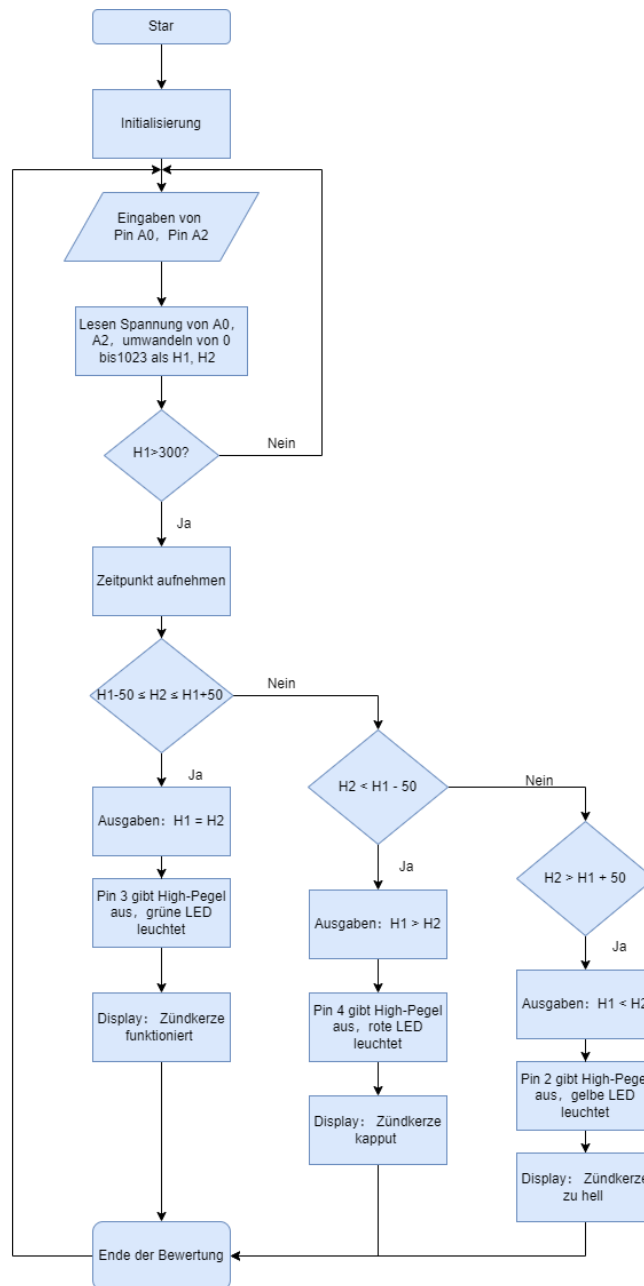
Abbildung 13: Ablaufdiagramm für Messverfahren
