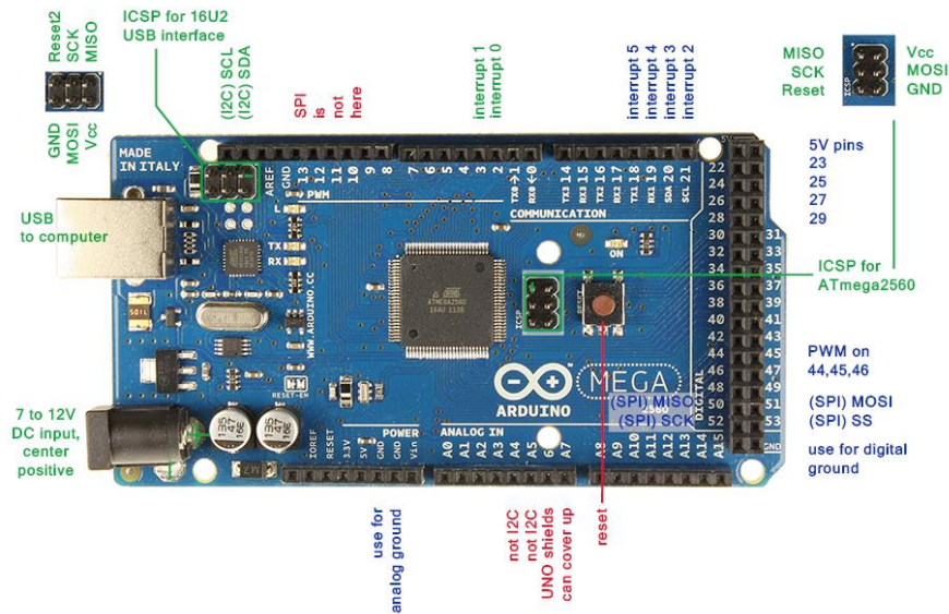
Abbildung 8:Arduino Mega 2560[4]
