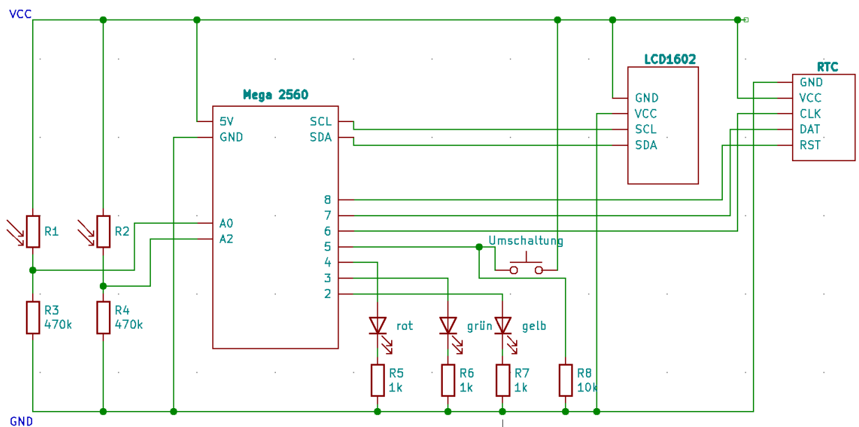
Abbildung 12:Schaltplan
