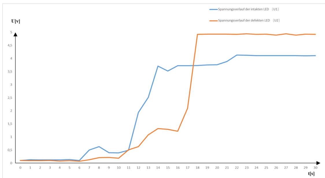
Abbildung 28: Spannungsverläufe der intakte LED (U1) und defekte LED (U2) beim Fall 3
