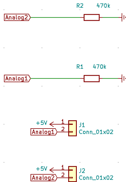
Abbildung 31: Schaltungsplan1
