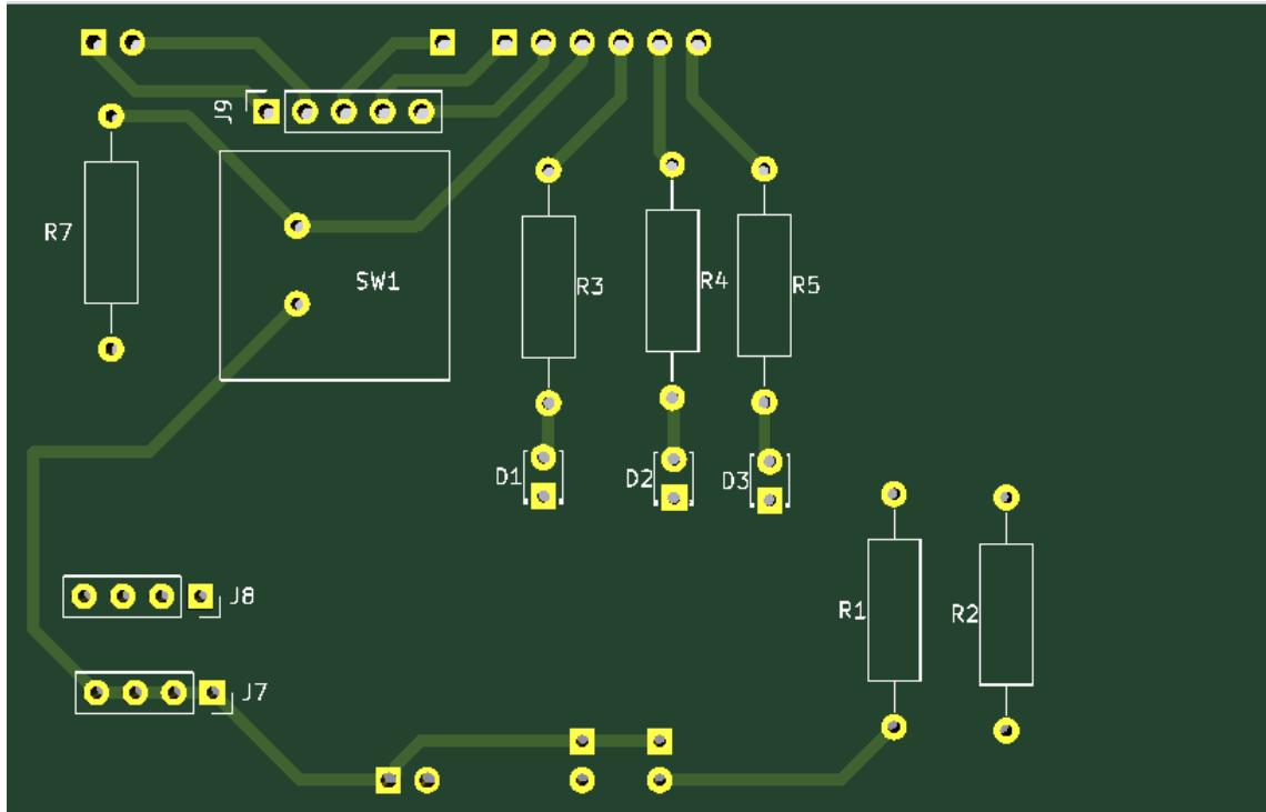
Abbildung 34: Abbildung 30: PCB(Vorderseite)
