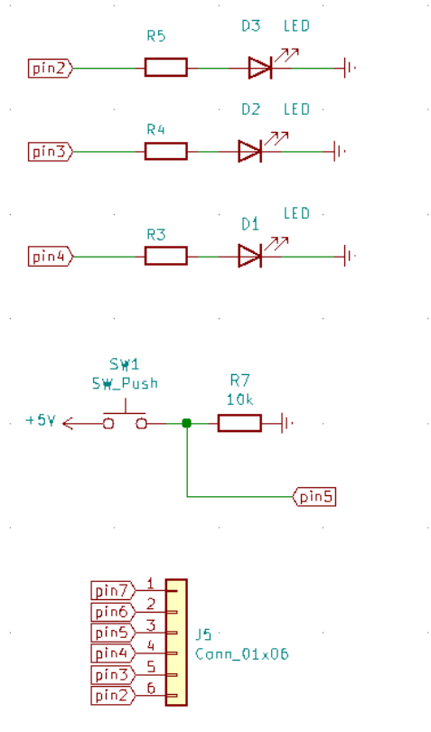
Abbildung 33: Schaltungsplan 3
