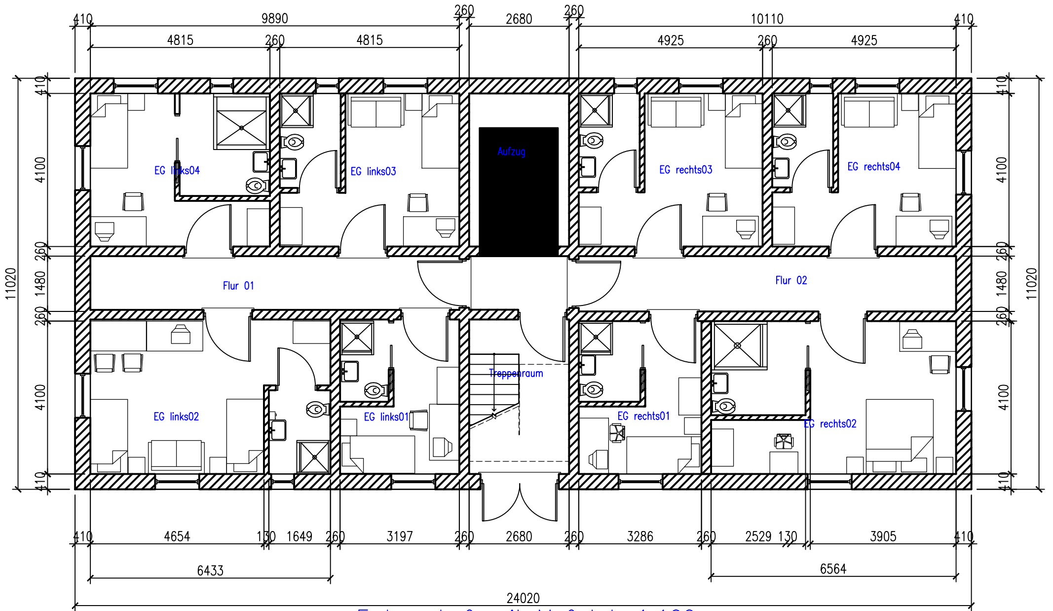
Erdgeschoß mit Maßstab 1:100
