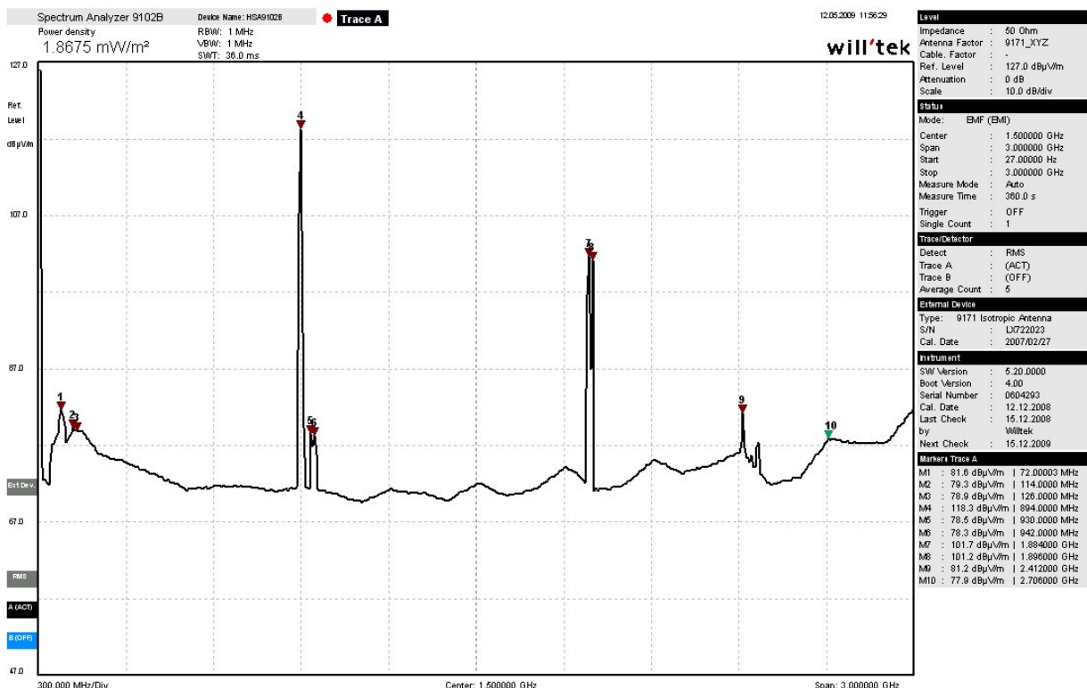
Abb.: Bild der frequenzselektiven HF Messung im Bereich 27 MHz bis 3 GHz.
