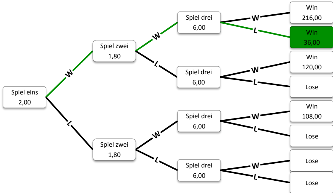
Abbildung 2: Systemwette „2 aus 3“ – Gewinnwege
