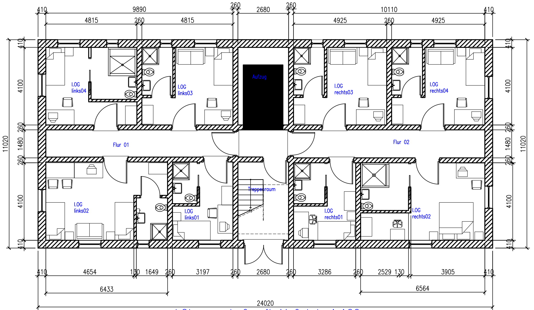
I.Obergeschoß mit Maßstab 1:100
