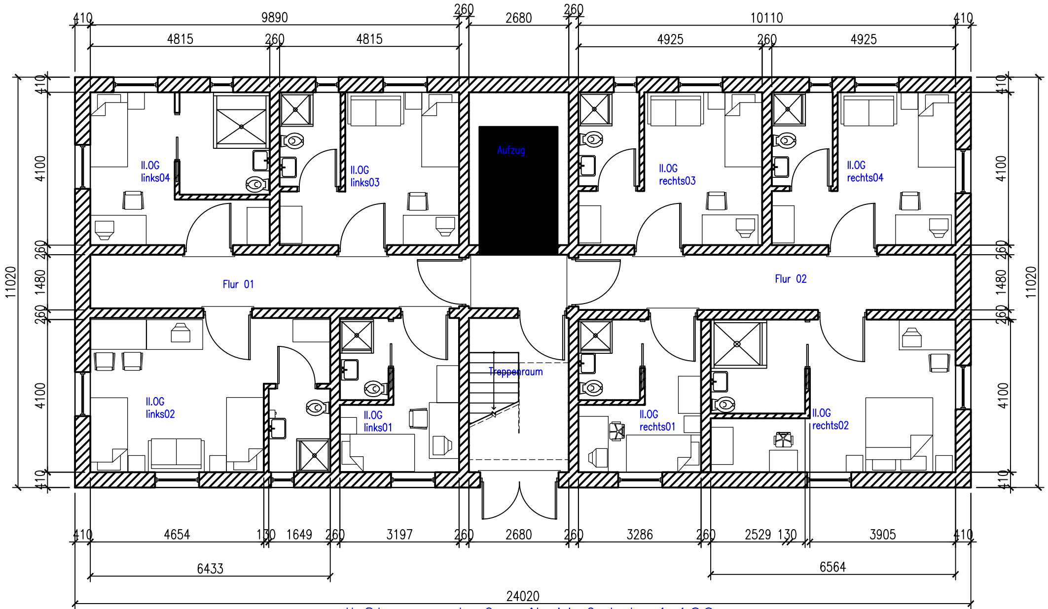
II.Obergeschoß mit Maßstab 1:100
