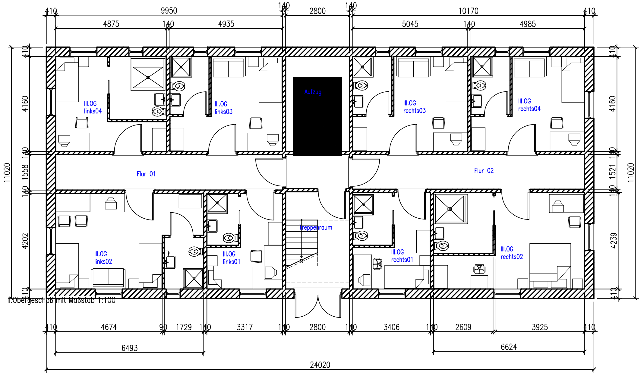
III. Obergeschoß mit Maßstab 1:100
