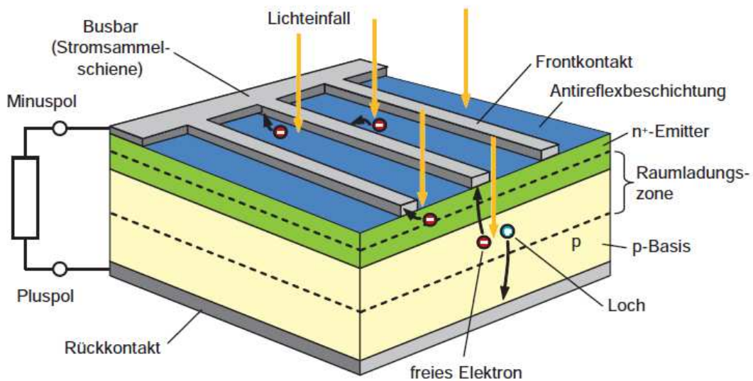
Abbildung 6: Typische Silizium-Solarzelle 70
